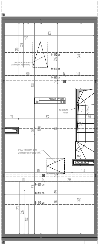
PODDASZE
