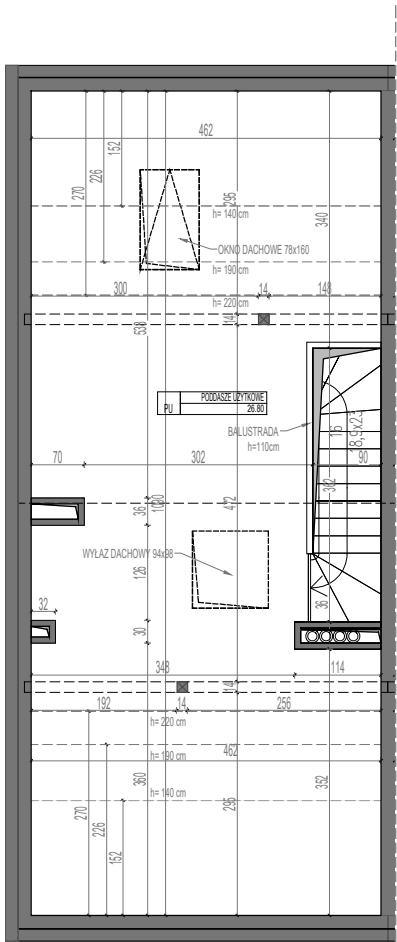
PODDASZE
